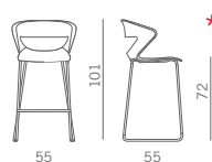
Telaio 4 gambe Versioni: AV AB AN ACC A richiesta altri colori telaio (min. 10 pz) 4 legs frame Versions: AV AB AN ACC Different frame finishes on request (min. 10 pcs)
