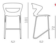
Telaio semi slitta Versioni: AV AB AN ACC Slope sled frame Versions: AV AB AN ACC
